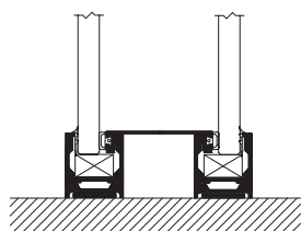
Gulvtilslutning
