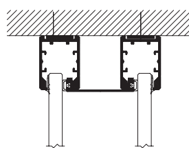
Lofttilslutning
