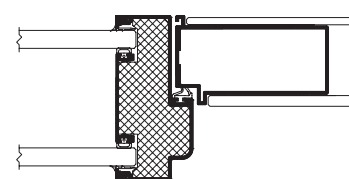
DG glasdør
