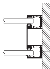
Vægttilslutning
