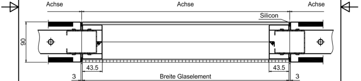
Schnitt A-A
