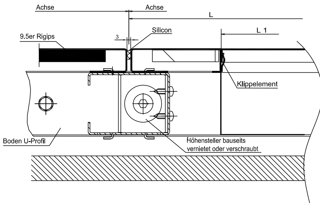
Ansicht
