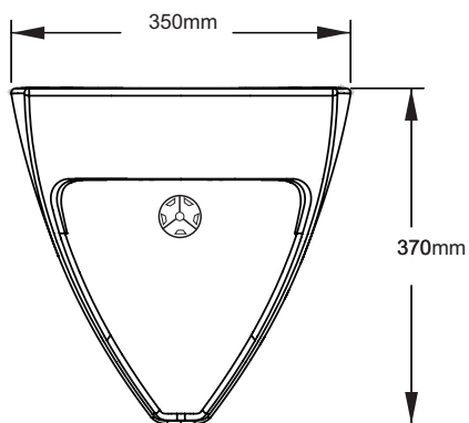
Frontansicht
